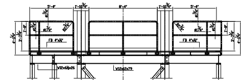
SECTION J-J.
